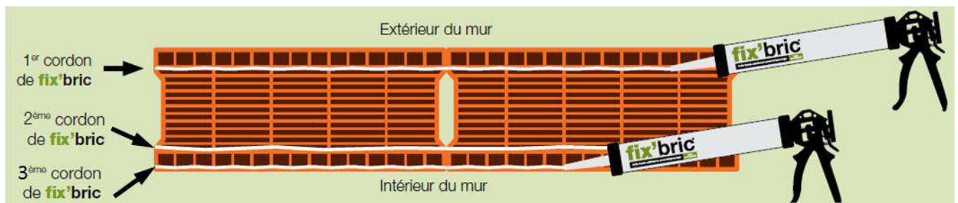
Figure 16 Pose du procédé fix'bric N dans les angles de murs
