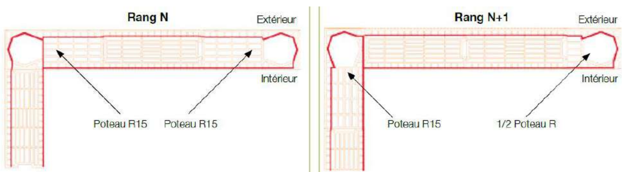
Figure 16 Pose du procédé fix'bric N dans les angles de murs
