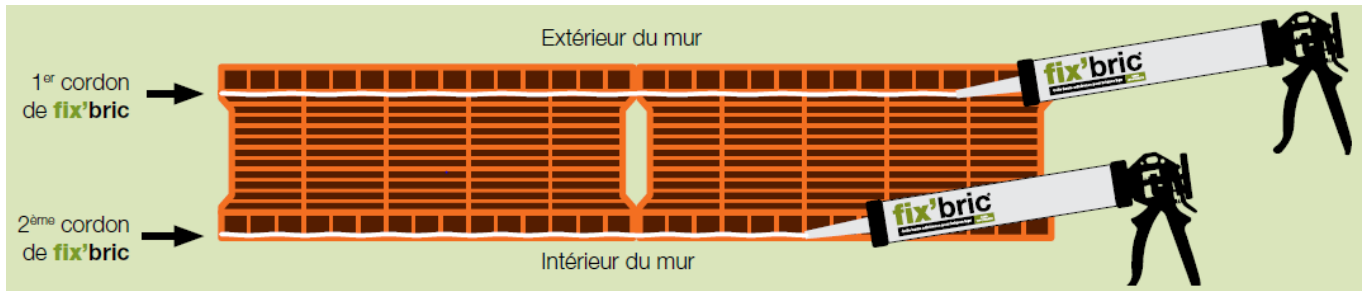
Figure 15 Pose du procédé fix'bric N - 3 cordons
