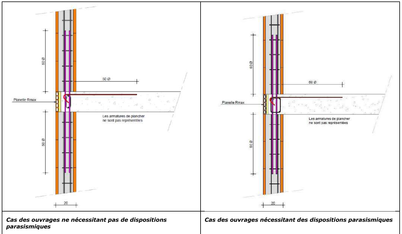
Figure 17 Coupe en about de plancher
