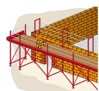
Échafaudage de pied
