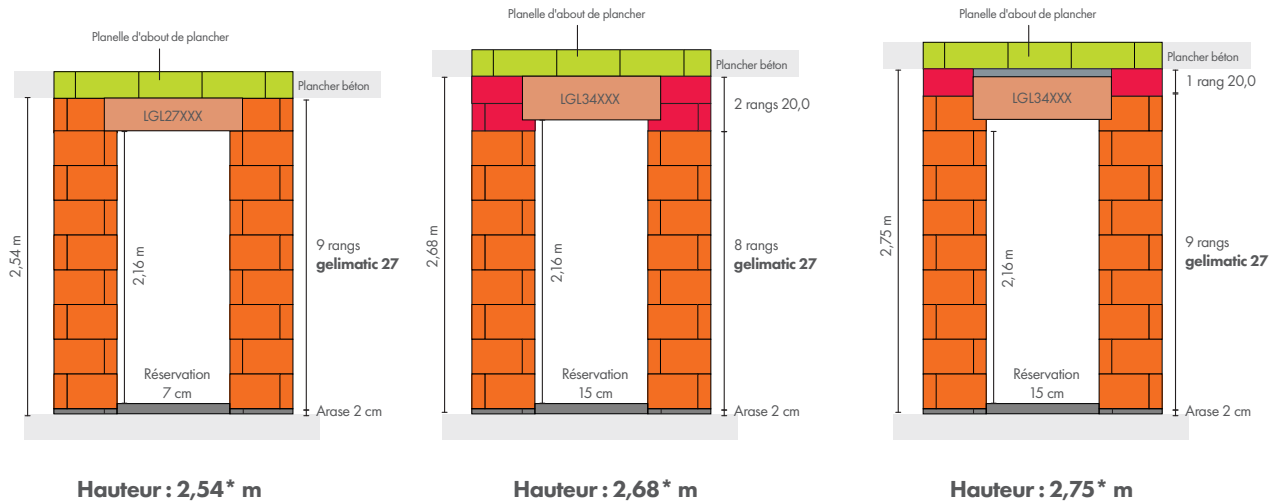
BRIQUE GELIMATIC 27 SCHÉMAS DE CALEPINAGES FRÉQUEMMENT UTILISÉS EN ÉLEVATION SOUS PLANCHER BÉTON
