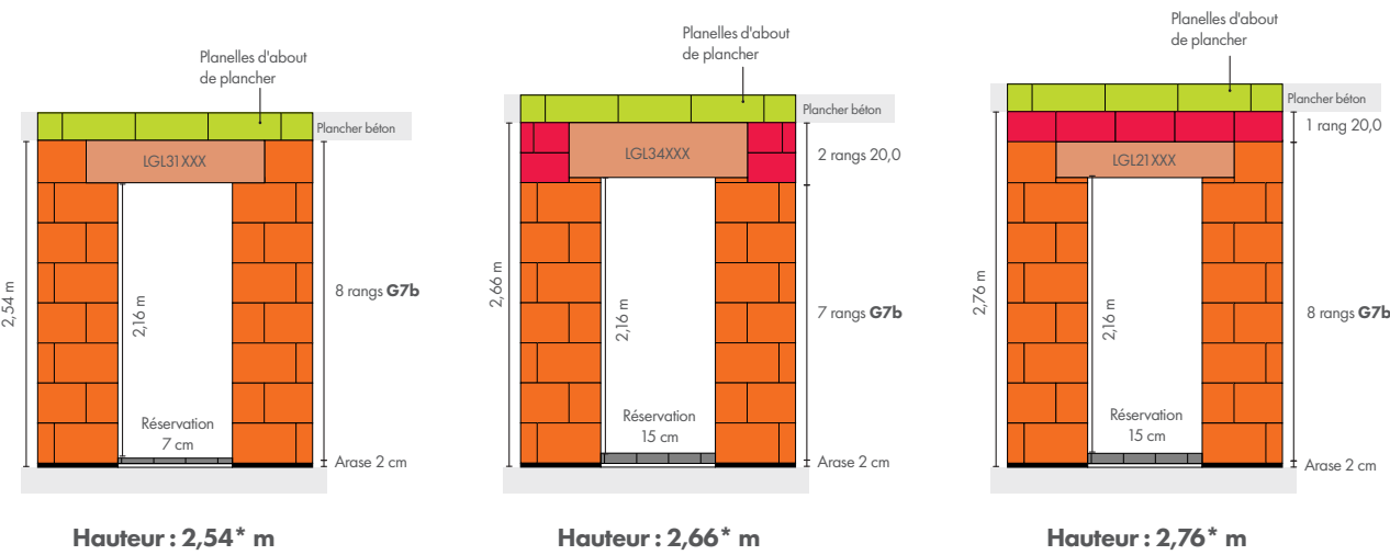
BRIQUE THERMO’BRIC G7B SCHÉMAS DE CALEPINAGES FRÉQUEMMENT UTILISÉS EN ÉLEVATION SOUS PLANCHER BÉTON
